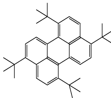
Tetra-tert-Butyl Perylene
