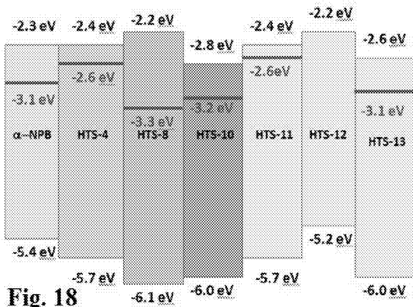
HOMO-LUMO values of HTs
